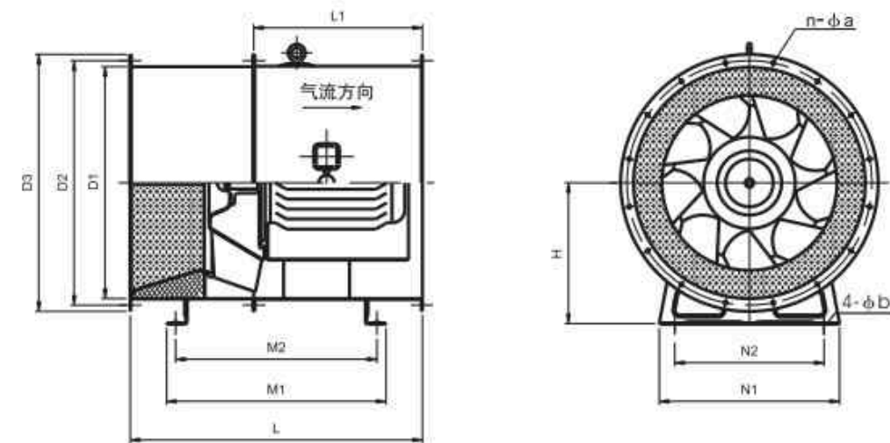
HL3-2A型混流风机外形及安装尺寸
