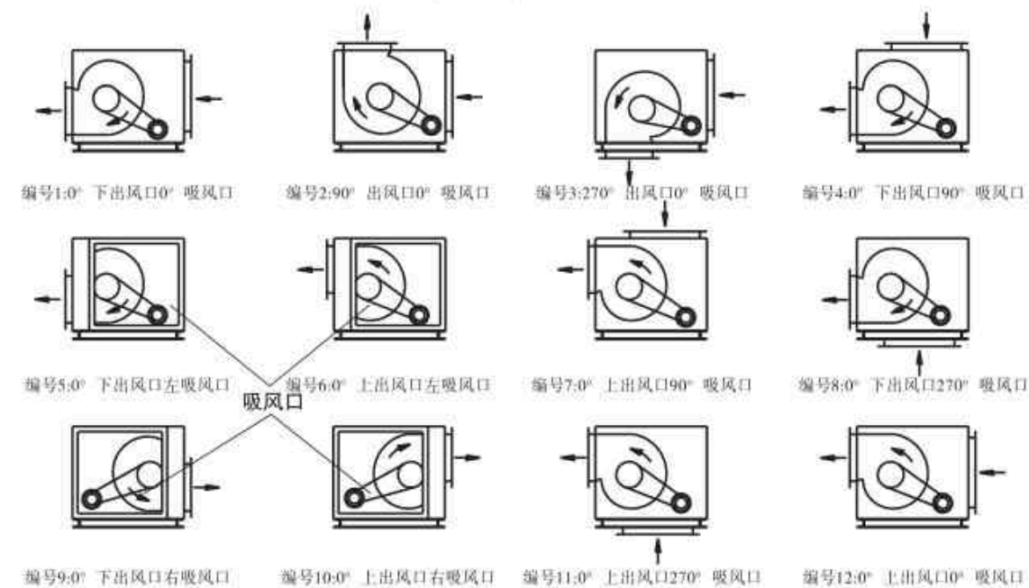
HTFC型柜式离心风机—B式
