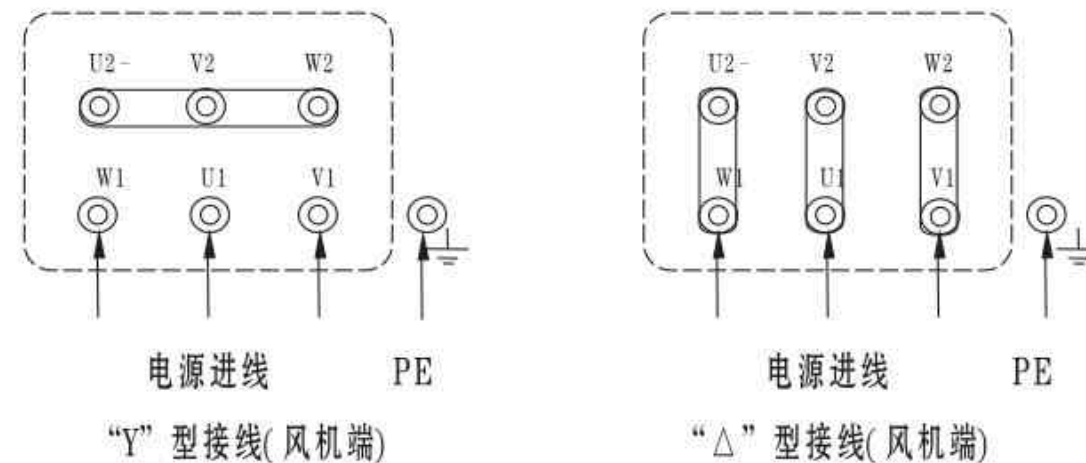
图6单速风机接线原理图
