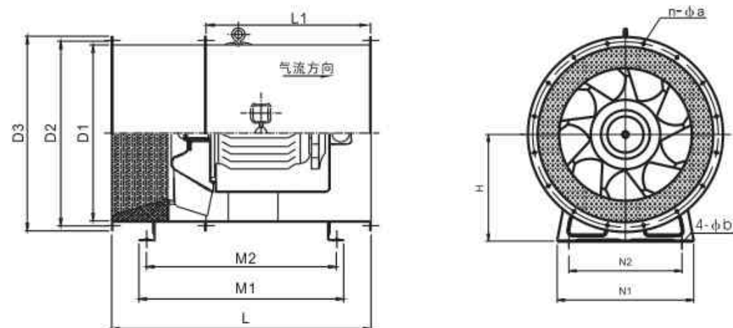
PYHL-14A型混流风机外形及安装尺寸
