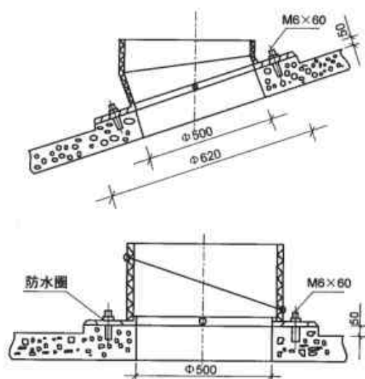
钢筋混凝土屋顶装设涡轮机(5 # )示意图 单位mm
