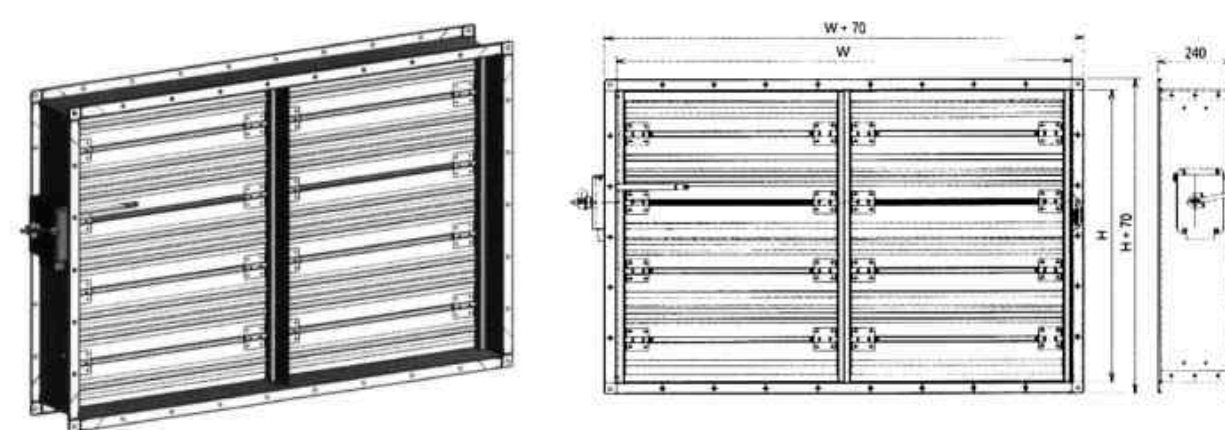
排烟阀外形结构图
