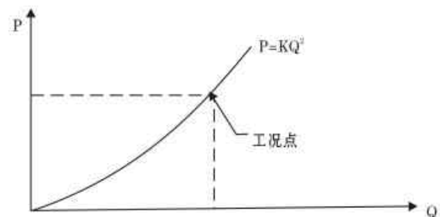
图2 系统阻尼曲线典型示例
