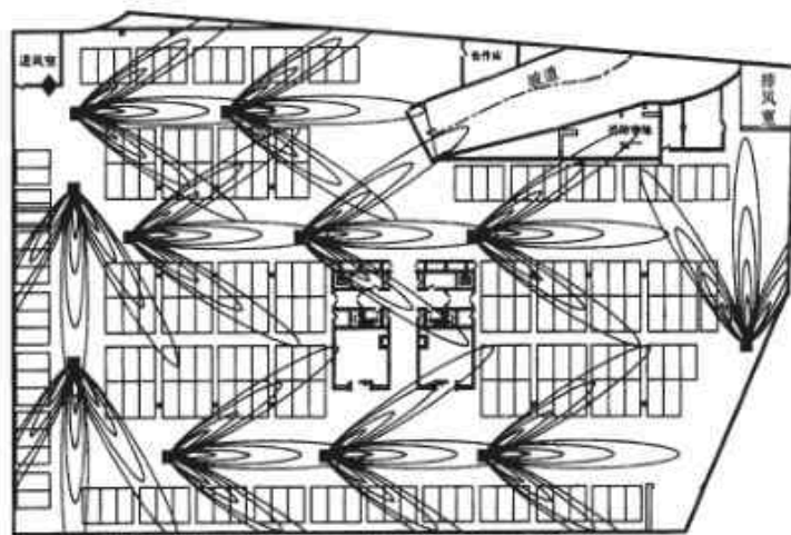
YDF诱导风机机组的配置及气流分布示意图
