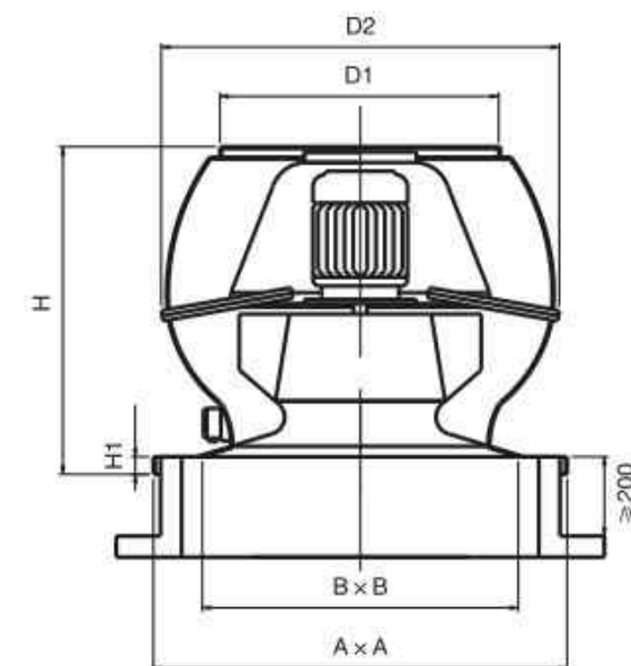
风机外形尺寸
