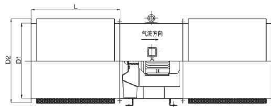
GXF-BX1消声型斜流风机安装尺寸表
