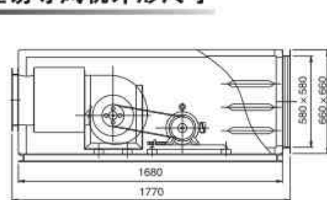
YDF-A-No2.5外形尺寸
