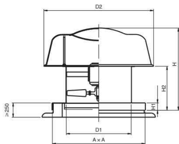
风机外形尺寸
