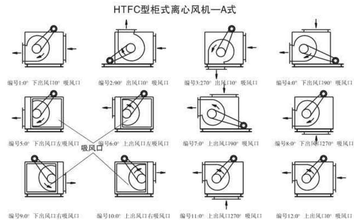
七、HTFC柜式离心风机封口位置图
