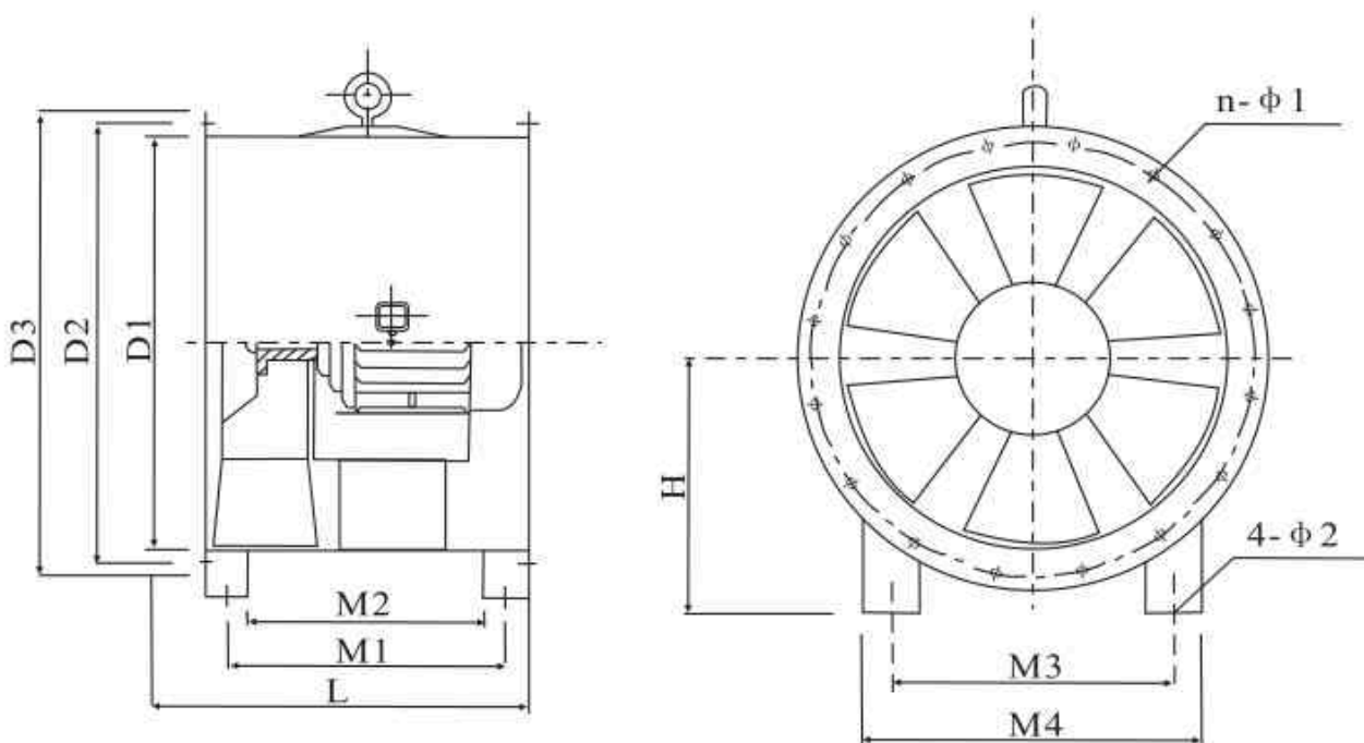
二、SDF型隧道式轴流风机外形及安装尺寸
