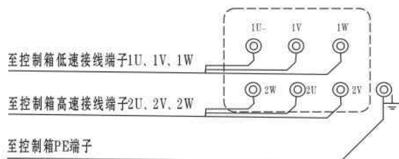
双速风机与双速控制箱连接接线图(风机端)
