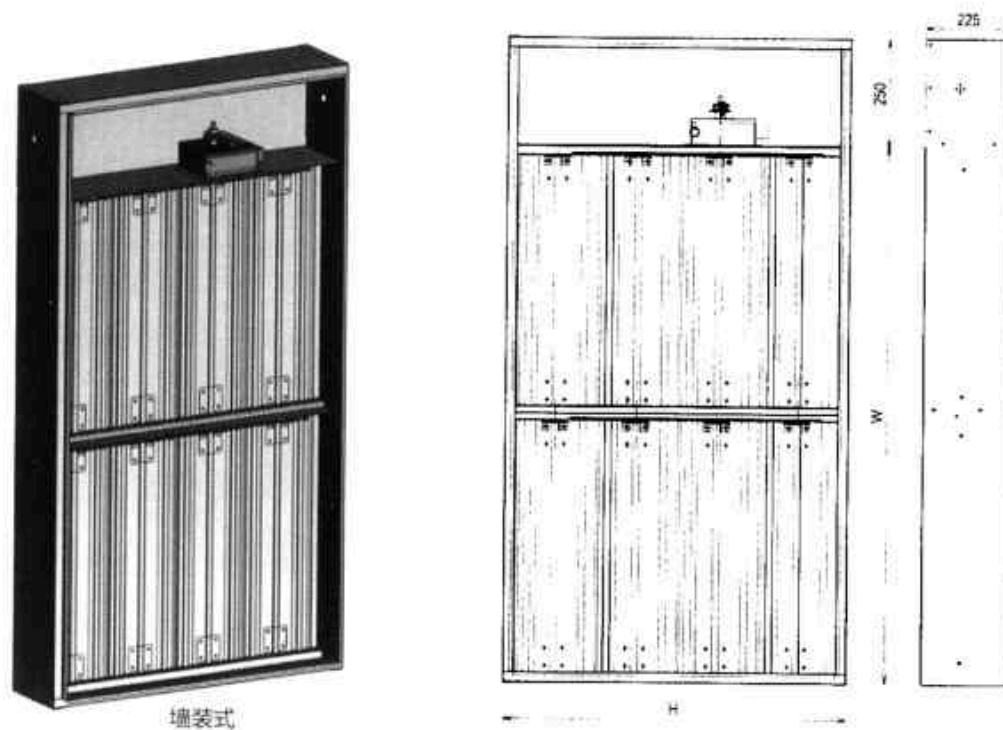
排烟阀外形结构图
