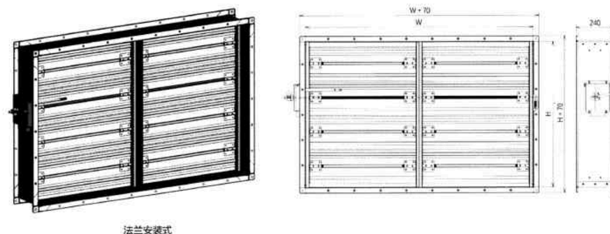
排烟防火阀外形结构图
