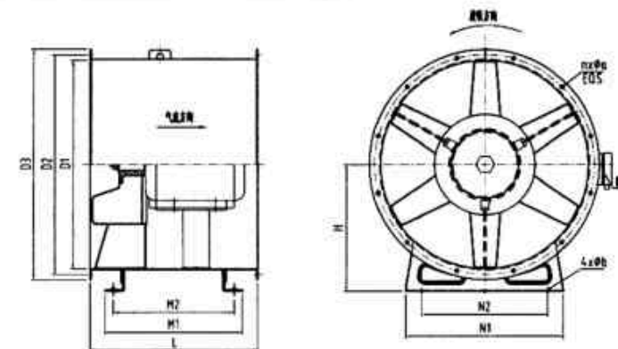
七、HTF-I 型轴流式消防排烟风机外形及安装尺寸
