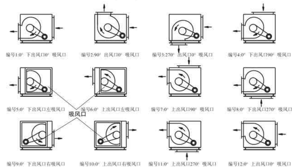
HTFC-B型柜式离心风机风口位置编号
