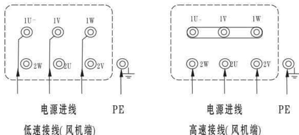
图7 单绕组双速风机接线原理图(不带控制箱)
