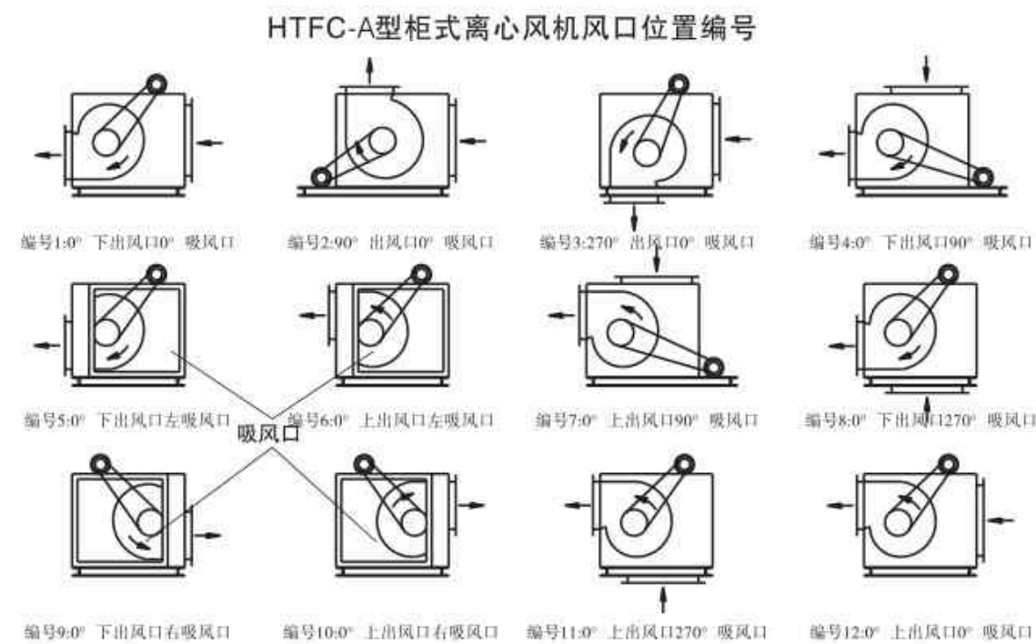
七、HTF-V柜式离心风机风机位置图
