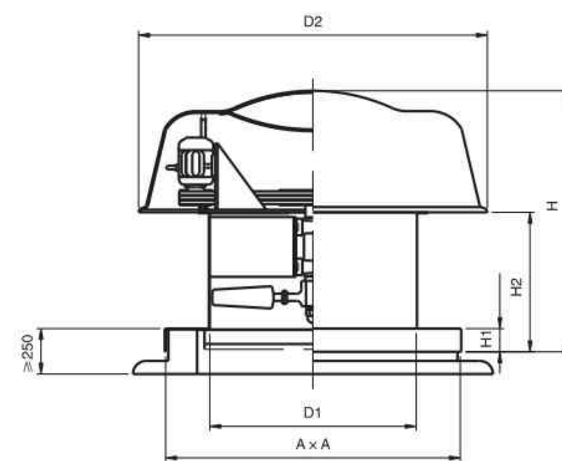
风机外形尺寸
