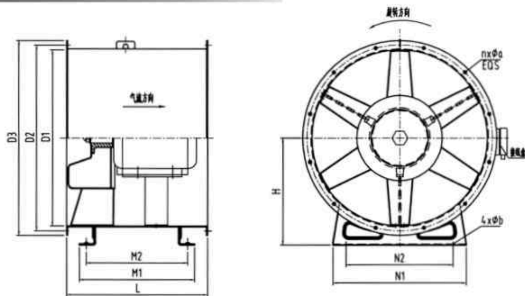
HTF-II 型轴流式消防排烟风机外形及安装尺寸
