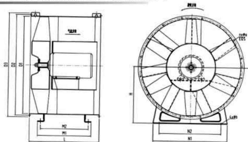
HTF-I 型轴流式消防排烟风机外形及安装尺寸
